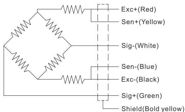
Wiring Code@Clockwise
